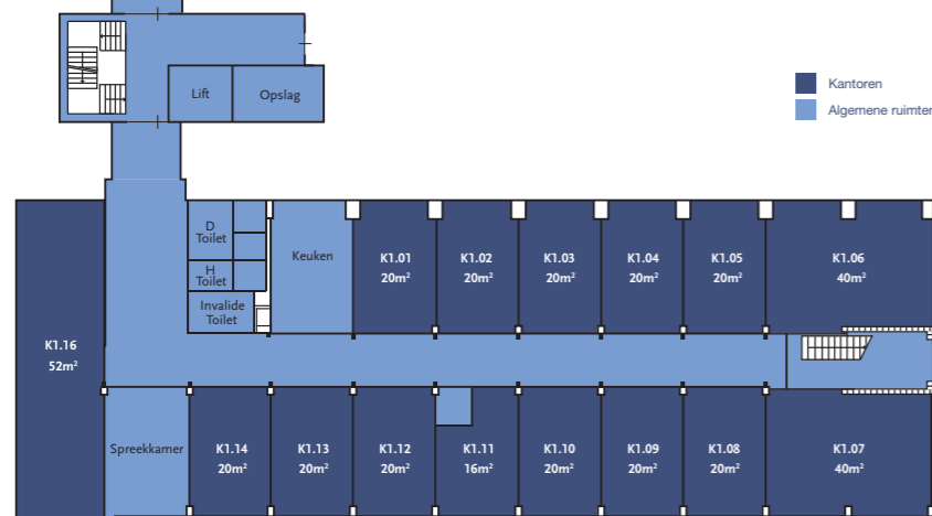
Eerste verdieping A-vleugel
